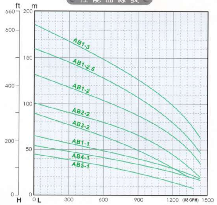
性能曲線表
