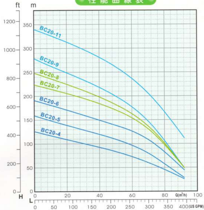
性能曲線表
