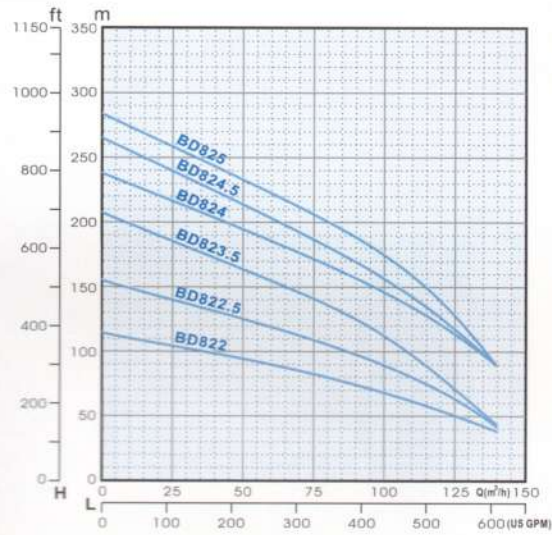
性能曲線表
