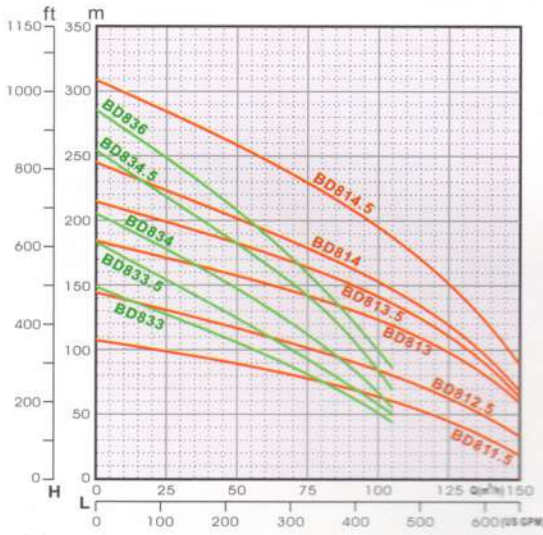
性能曲線表
